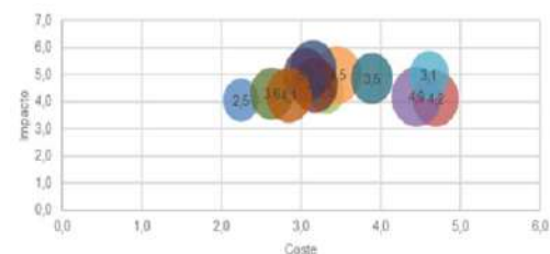
Ilustración 132. Matriz Coste-Impacto-Factibilidad
