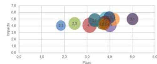
Ilustración 134. Matriz Plazo-Impacto-Coste
