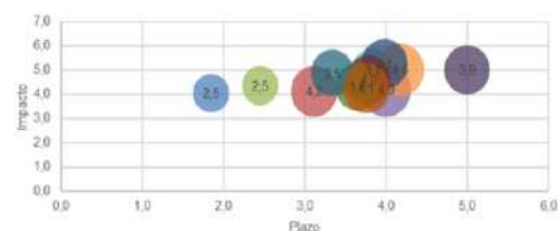
Ilustración 135. Matriz Criticidad-Impacto-Reiteración
